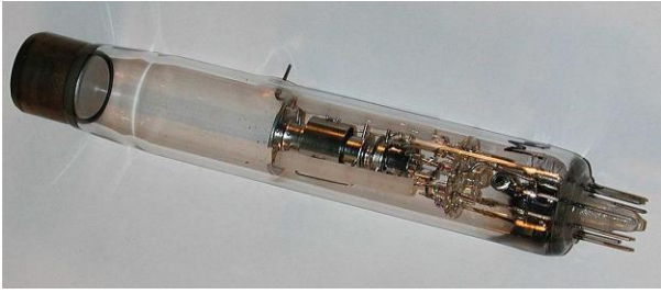
Fot. 9 Lampa rentgenowska z anodą transmisyjną [9]
