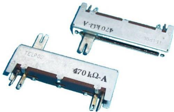
Fot. 12 Potencjometr suwakowy [9]
